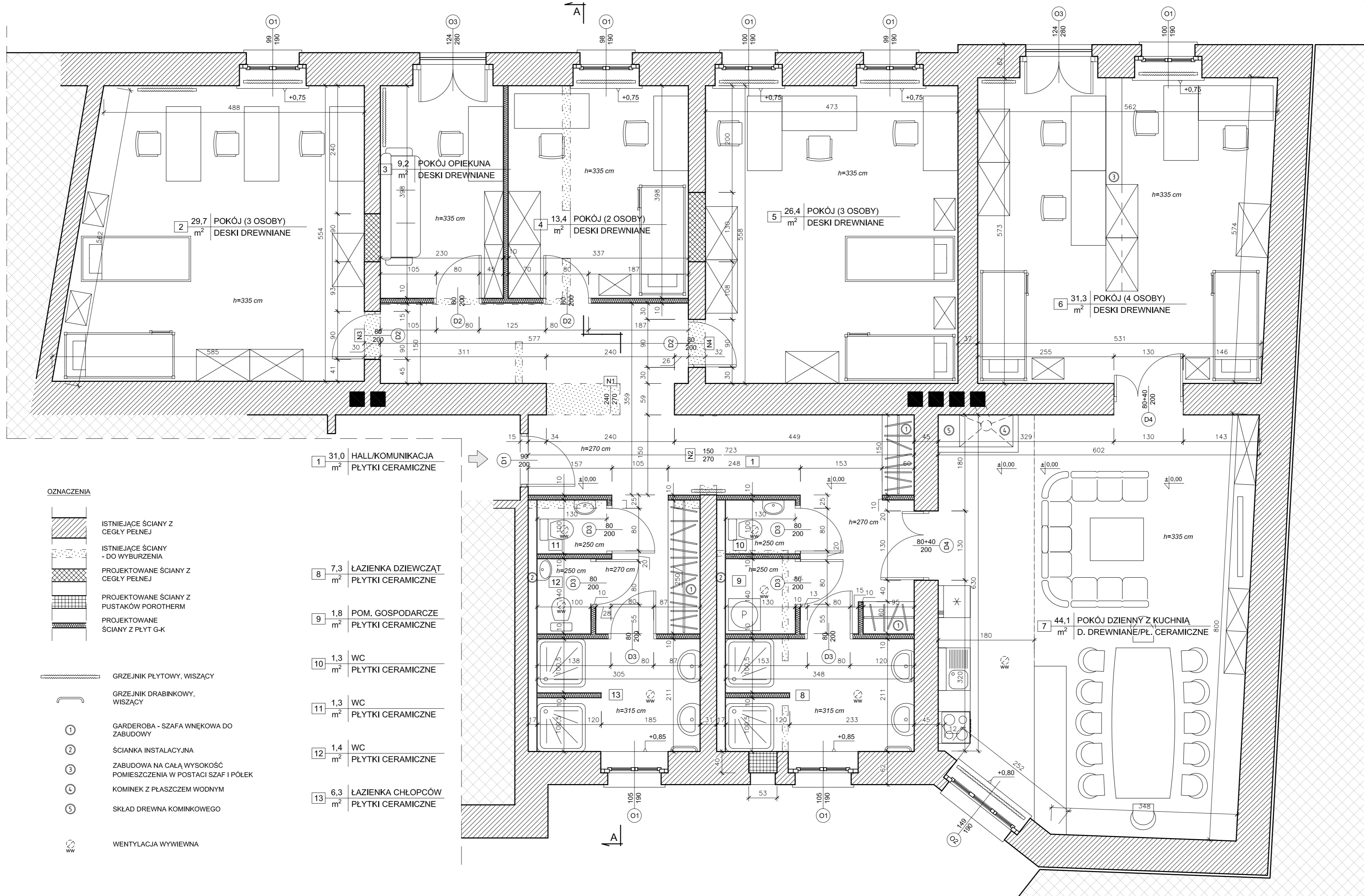
PROJEKT PRZEBUDOWY - RZUT SKALA 1:50
